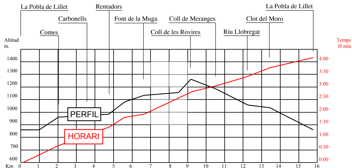
PERFIL I HORARI. ANY 2013
